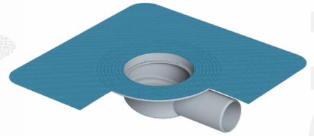
Su Yalıtımlı Yatay Çıkış / Waterproof-Horizontal Outlet Ø32 - Ø50 - Ø70 - Ø100
